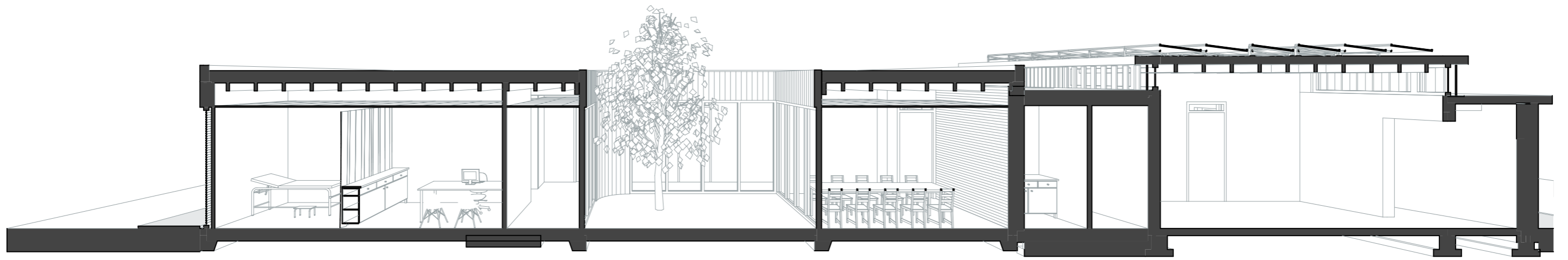
Doorsnede B2
