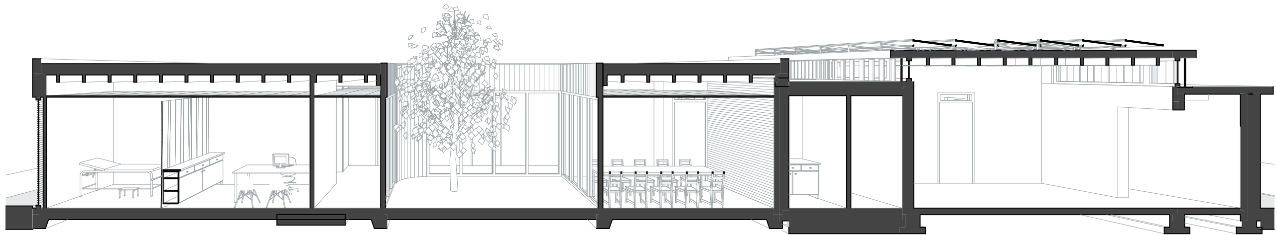
Doorsnede B2
